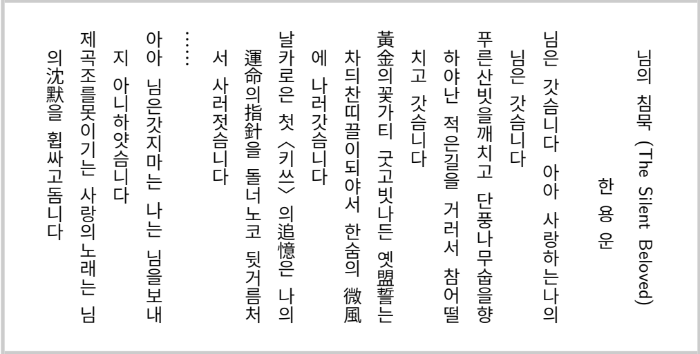
그림 2: 세로쓰기 보기. Noto Sans CJK KR 글꼴을 이용했다. 이 글꼴의 세로쓰기 어간이 1em으로 매우 커서 \spaceskip=0.5em plus.25em minus.125em 을 강제했다. CharRaise=.5ex 도 글꼴 옵션에 추가했다. 또한 \latinparens 를 선언했는데 제목 다음의 괄호가 CJK 괄호가 아니라 아스키 괄호이기 때문이다.
