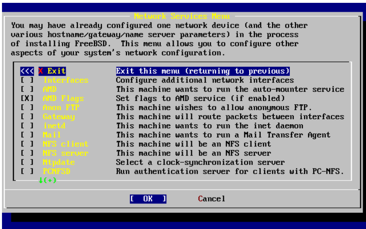
Рисунок 54. Верхняя часть меню настройки сети (Network Configuration)
