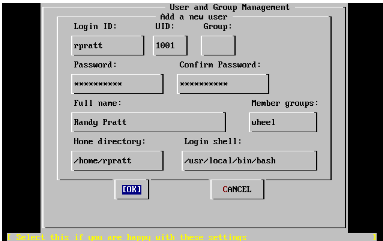
Рисунок 51. Ввод информации о пользователе
