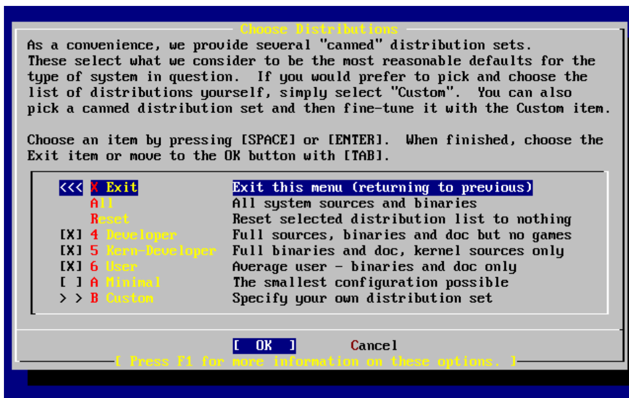
Рисунок 25. Подтверждение выбора дистрибутивного набора
