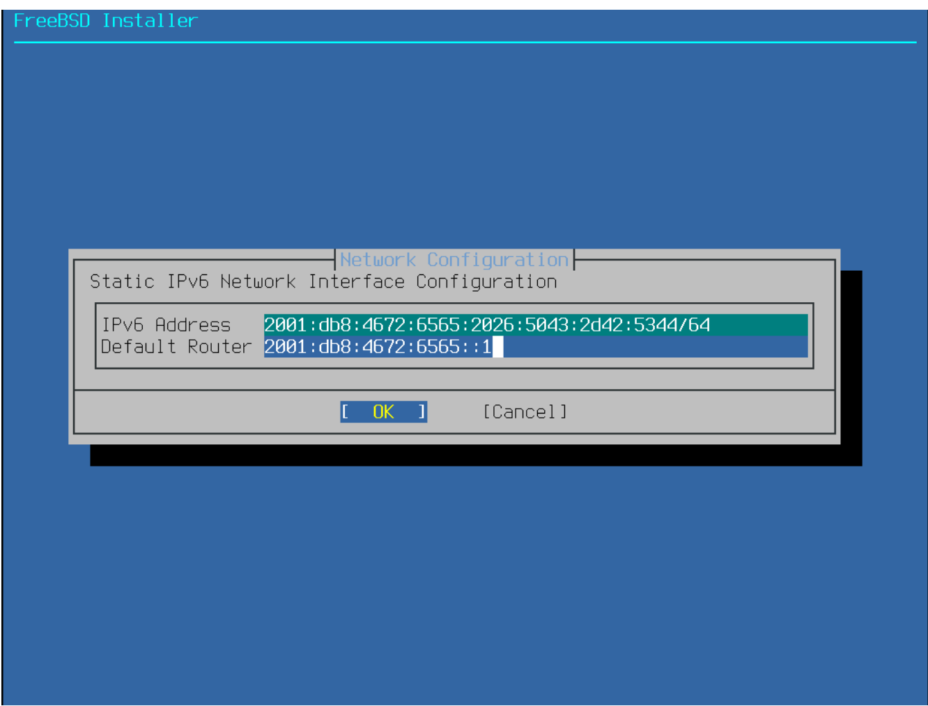
Рисунок 87. Статическая настройка протокола IPv6
