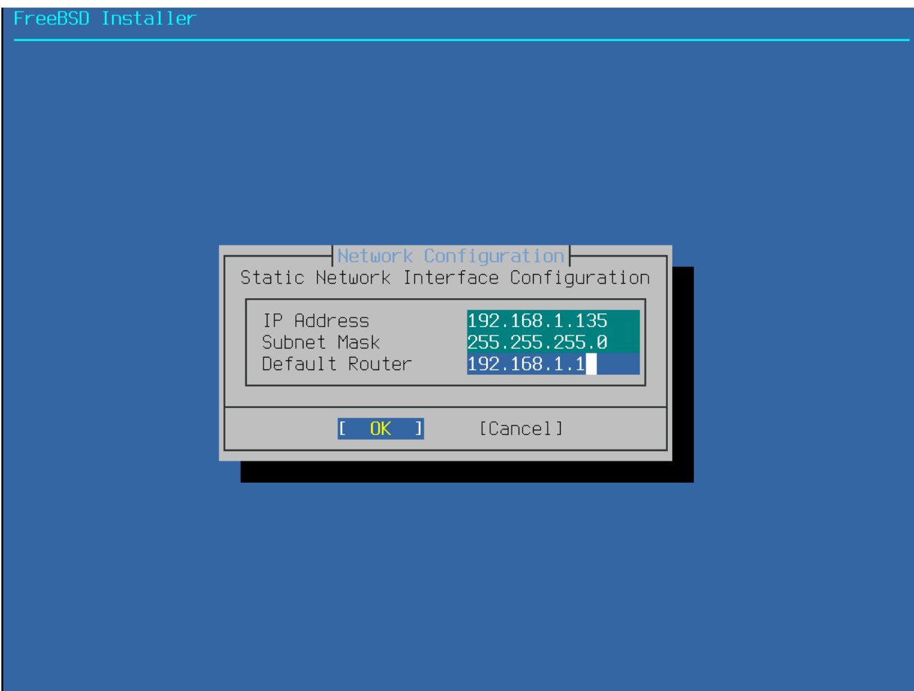
Рисунок 84. Статическая настройка IPv4 на сетевом интерфейсе
