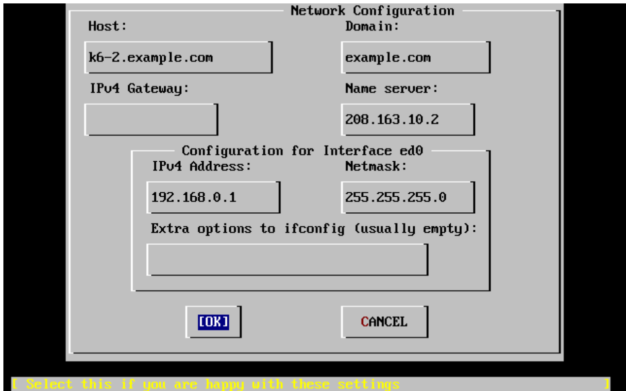
Рисунок 28. Настройка сети для ed0
