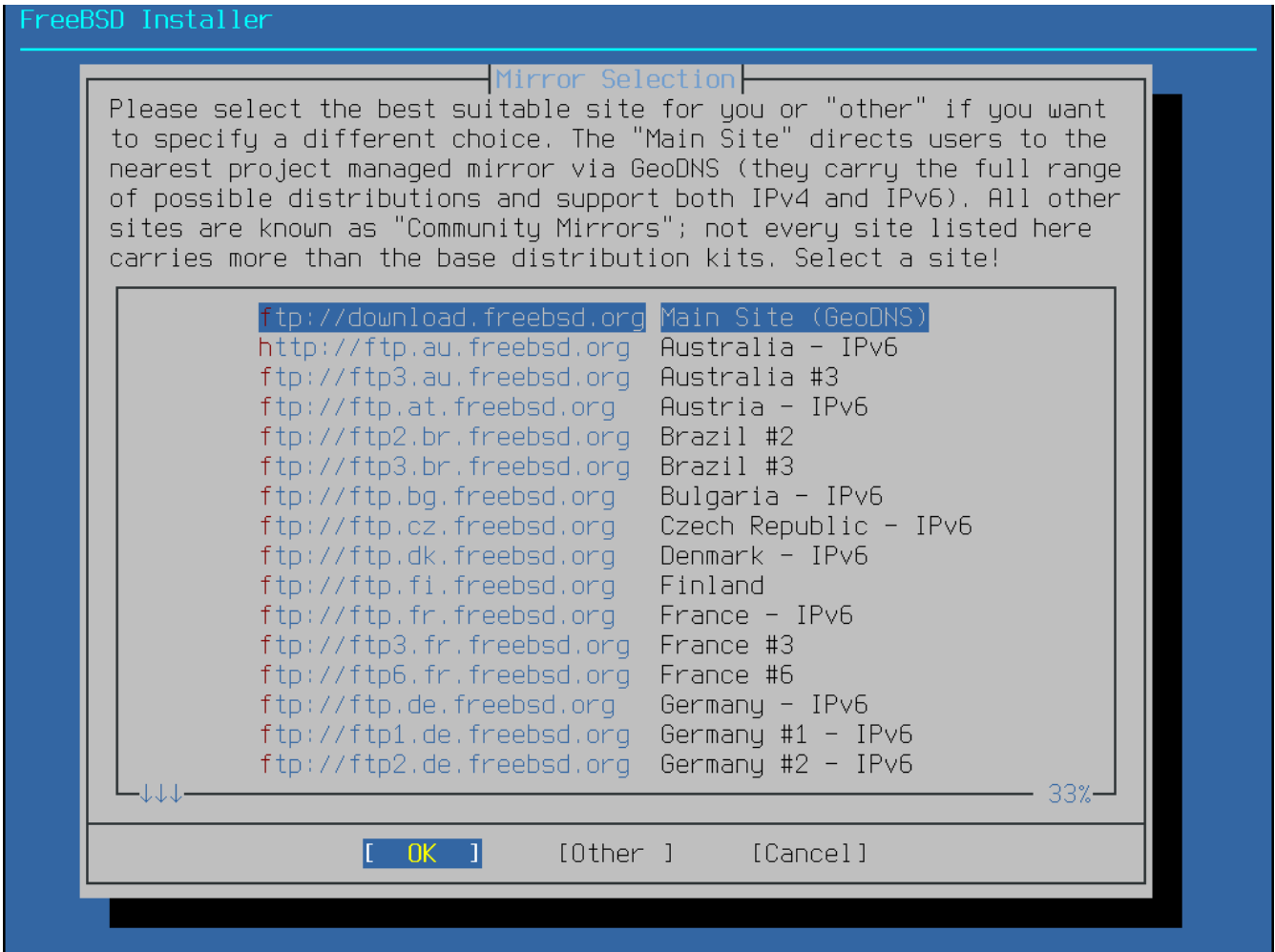
Рисунок 65. Выбор зеркала сайта
