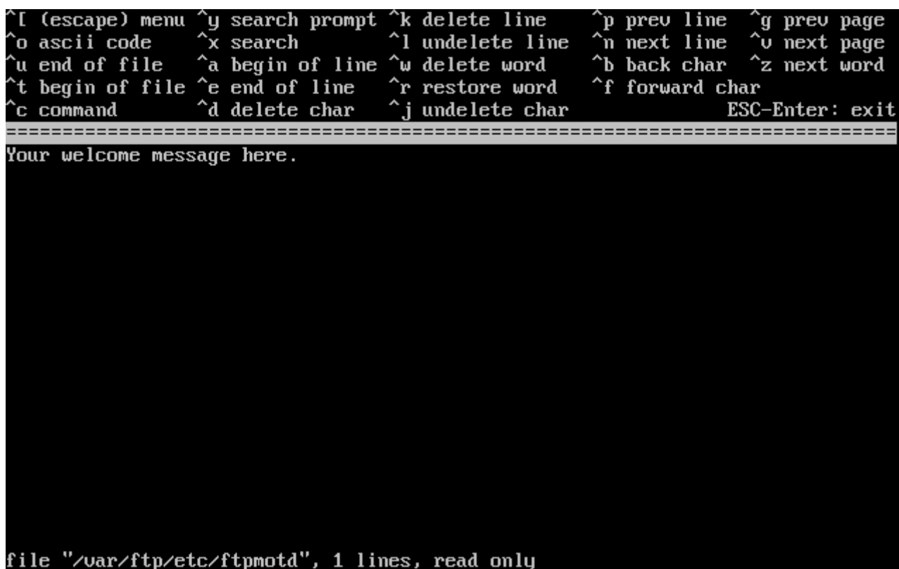
Рисунок 31. Редактирование FTP Welcome Message
