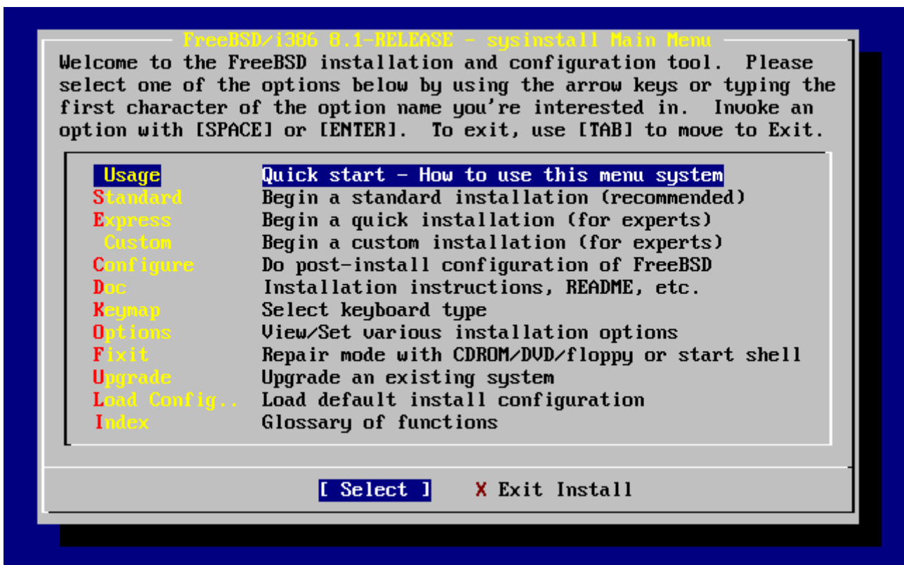
Рисунок 4. Выбор Usage в главном меню Sysinstall
